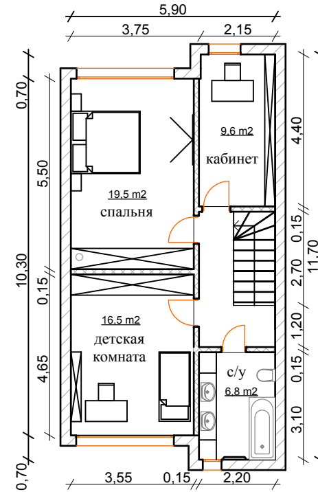
3 этаж 63,8 м 2
