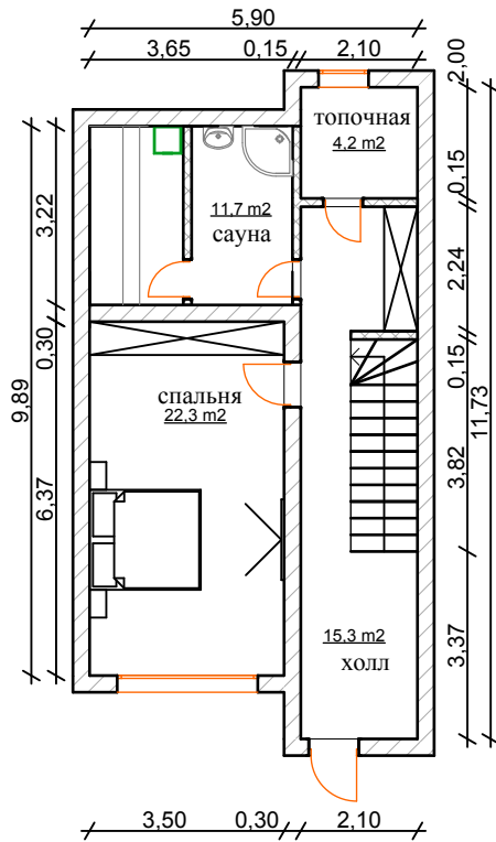
1 этаж 62,3 м 2
